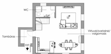
Buto patalpų išdėstymo planas 1 aukštas
