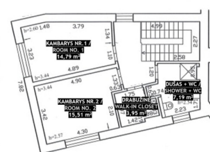
2 AUKŠTO PLANAS / GROUND FLOORPLAN
