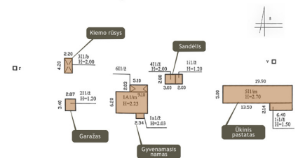
STATINIŲ IŠDĖSTYMO PLANAS
