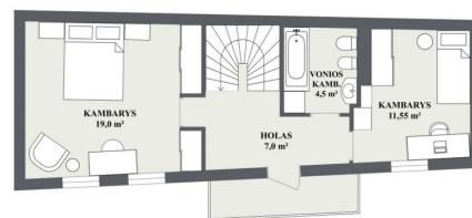
ANTRAS AUKŠTAS
