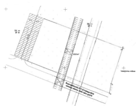
ZEMES SKLYPO PLANAS M 1:500 Sklypo plotas 3091 m 2
