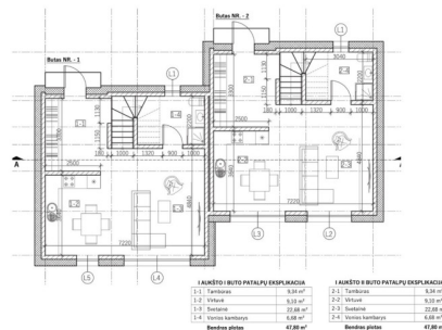
1 aukštas
