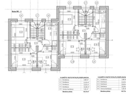
2 aukštas
