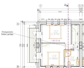
ANTRO AUKŠTO PLANAS SU NUMATOM
