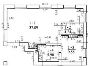
PIRMO AUKŠTO PLANAS PIRTIES PASTATAS
