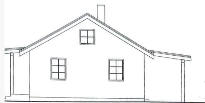
ŠONINIS (ŠR) FASADAS
