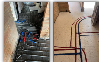
Išvedžiotas grindinis šilūymas
