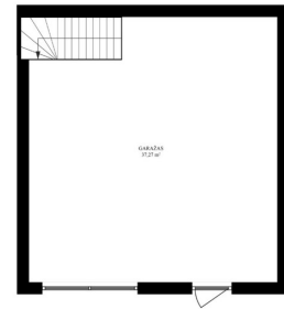
GARAŽO PLANAS PLOTAS - 17,27 m 2
