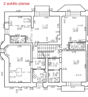
2 aukšto planas
