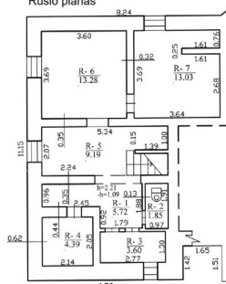
Rūsio planas
