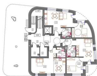
PIRMO ALKŪSTO PLANAS M1:100
