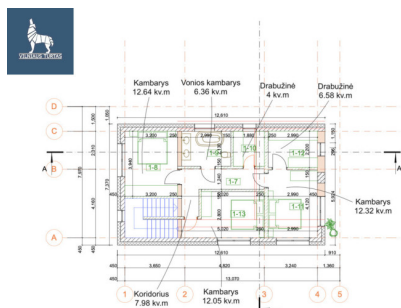
Suprojektuoto namo išplanavimas | II aukštis
