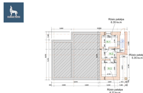
Suprojektuoto namo išplanavimas | rūšys
