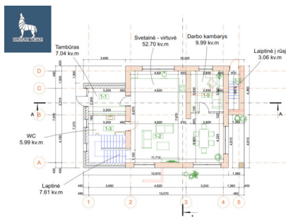
Suprojektuoto namo išplanavimas | I aukštis
