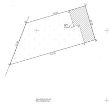
ŽEMES SKLYPO PLANAS M 1:500 Žemės sklypo plotas 1361 m 2
