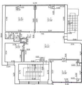
TREČIAS AUKŠTAS
