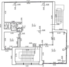
KETVIRTAS AUKŠTAS
