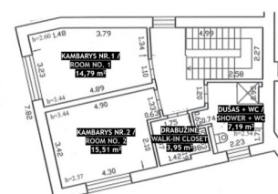
2 AUKŠTO PLANAS / GROUND FLOORPLAN
