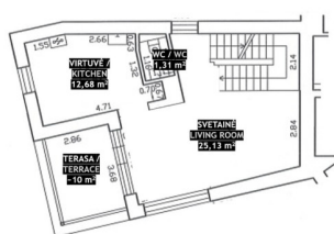
1 AUKŠTO PLANAS / 1 FLOORPLAN
