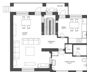
PIRMAS AUKŠTAS
