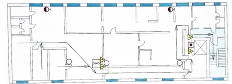
II AUKŠTO PATALPŲ PLANAS Bendras plotas: 406,52 kv.m.
