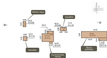
STATINIŲ IŠDĖSTYMO PLANAS
