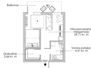
Buto patalpų išdėstymo planas Bendras plotas - 37,18 kv. m
