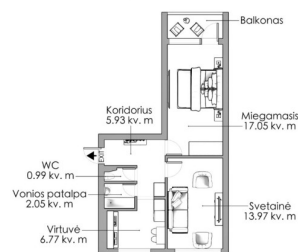
Buto patalpų išdėstymo planas Bendras plotas - 46.76 kv. m
