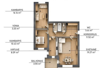
3 KAMBARIŲ BUTO PATALPŲ EKSPLIKACIJA BENDRAS PLOTAS - 73.66 m 2
