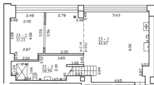
BUTO PLANAS 1 aukštas
