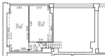
BUTO PLANAS 2 aukštas
