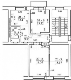
Antras aukštas
