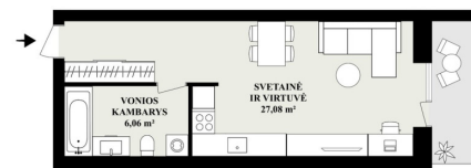
IŠPLANAVIMAS BENDRAS PLOTAS - 33,14 m 2
