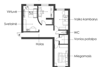
Buto patalpų išdėstymo planas Bendras plotas - 66 kv. m
