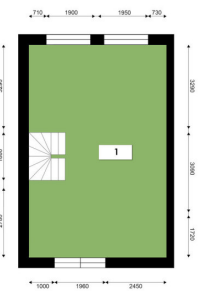
3 aukšto planas
