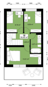
2 aukšto planas
