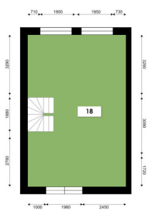
3 aukšto planas
