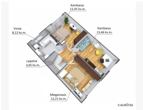
II AUKŠTAS
