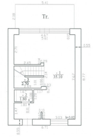
Pirmo aukšto planas
