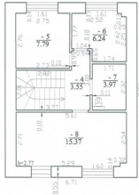
Antro aukšto planas
