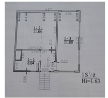
I aukštas
