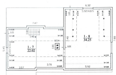
Pastogės planas
