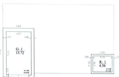
Rūsio planas
