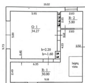
Rūsio planas
