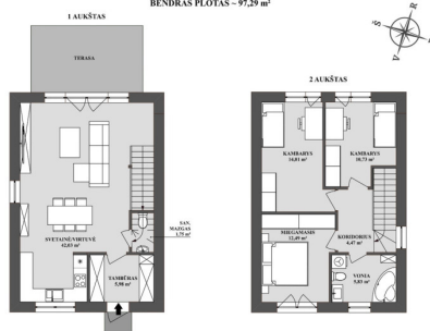
"A" BUTO PATALPŲ EKSPLIKACIJA BENDRAS PLOTAS - 97,29 m 2
