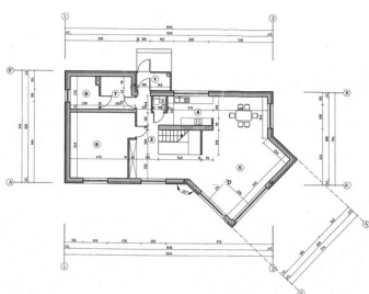
Pirmo aukšto plans
