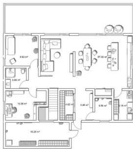
Pirmas aukštas
