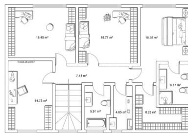
Antras aukštas
