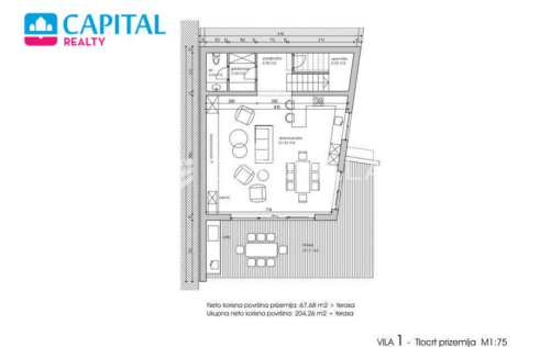
VILA 1 - I. kat - prizemlje M1:75
