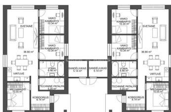
87 kv. m NAMŲ PLANAI
