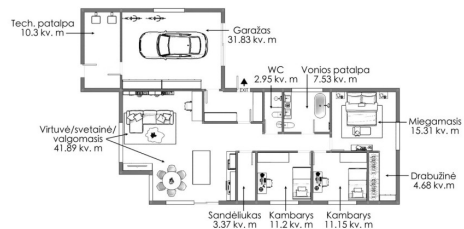
Namo patalpų išdėstymo planas
