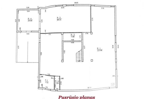
Pusrūsio planas
