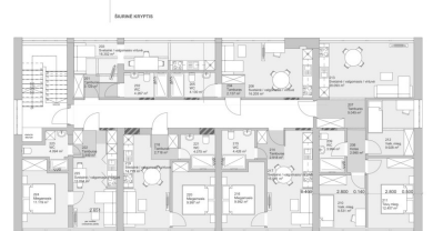
Antro aukšto planas M 1 : 100
