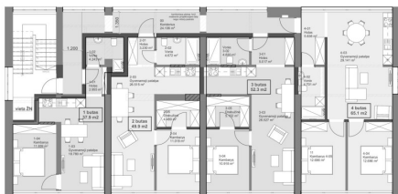
Butas A Butas B Butas C Butas D Antro aukšto planas M 1 : 100
