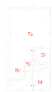
PATALPŲ PLANAS
