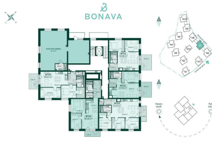
LAKE TOWN 147 KORPUSĀS PIRMO ALKSTO PLĀNS Eidžiņģu i., Vīķi
