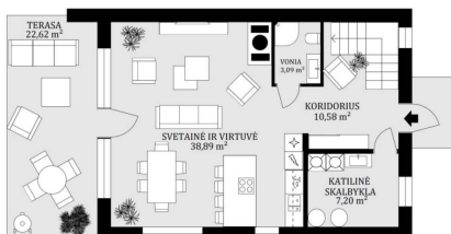
PIRMO AUKŠTO PATALPŲ EKSPLIKACIJA BENDRAS AUKŠTO PLOTAS - 59,76 m 2
