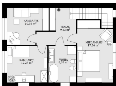
ANTRO AUKŠTO PATALPŲ EKSPLIKACIJA BENDRAS AUKŠTO PLOTAS - 58,28 m 2
